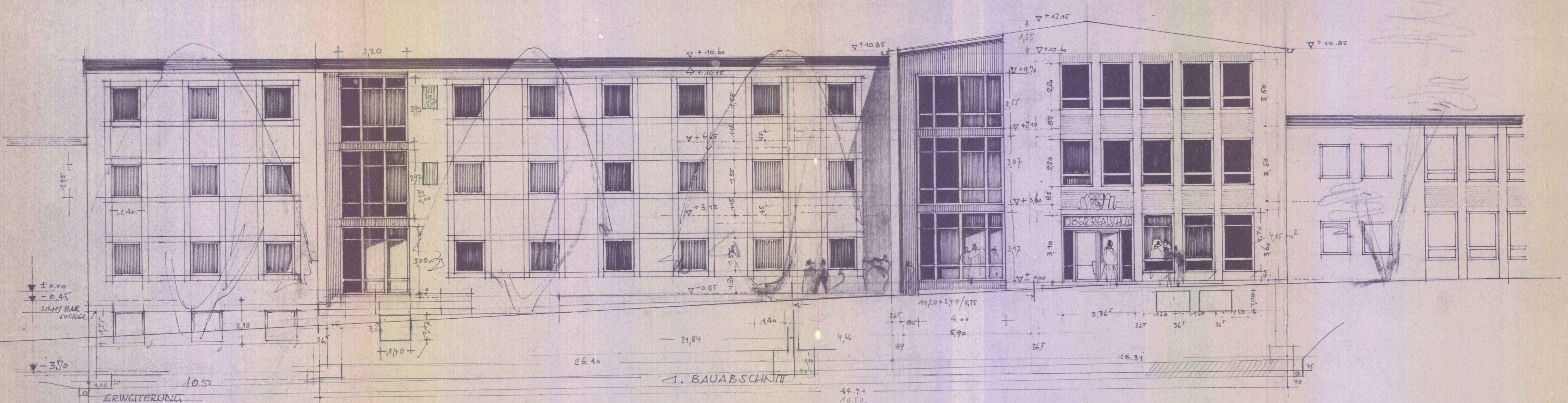
ANSICHT VON NORDEN VON DER VIMY-STRASSE AUS
